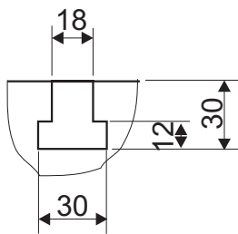
Detail A DIN650(ISO299)
